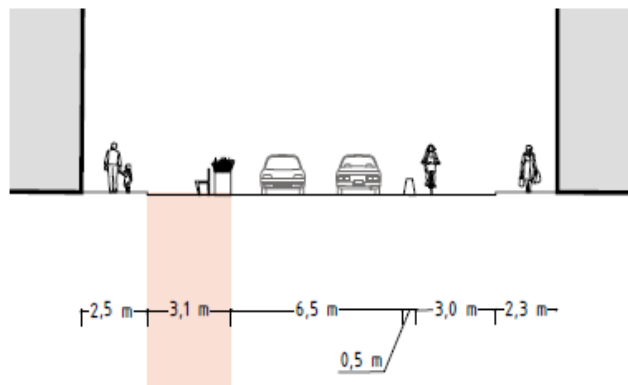
Periaatepoikkileikkaus 1:1000
